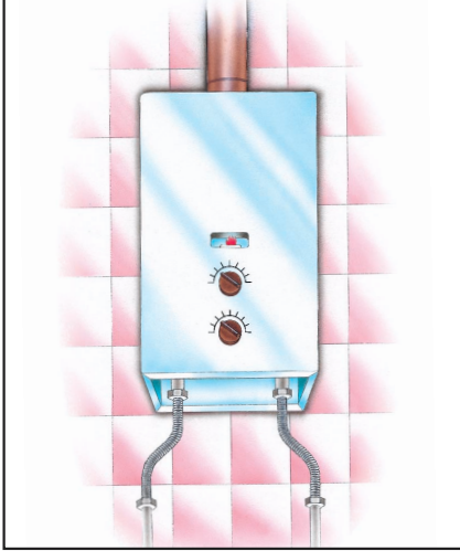
Şofben: Gaz giriş, sıcak su, soğuk su giriş ve çıkış bağlantıları. Water heaters: Natural gas inlet, cold water inlet, hot water inlet-outlet connections.
